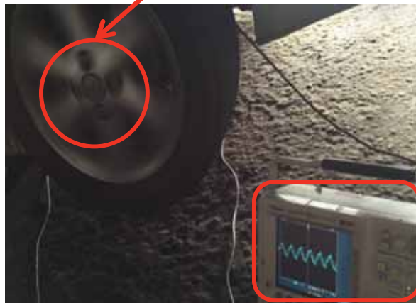
輪齒波形訊號擷取
